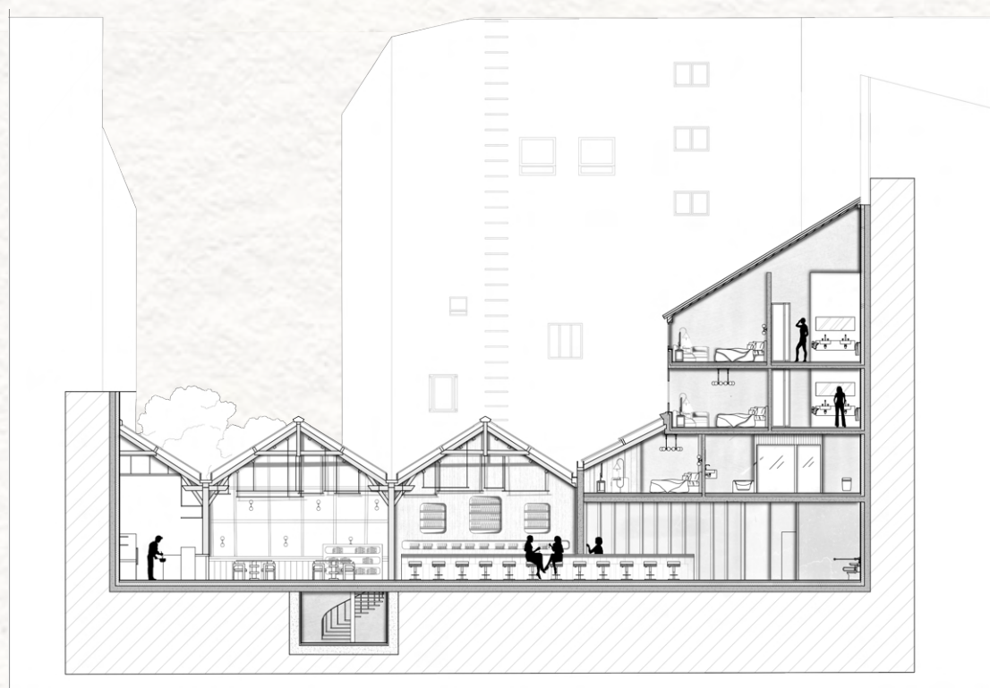
COUPE GÉNÉRALE DU BÂTIMENT
