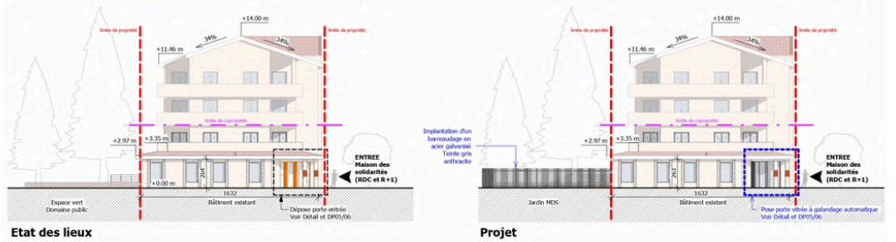
DP04 PLAN DE FACADE NORD Ech : 1/200
