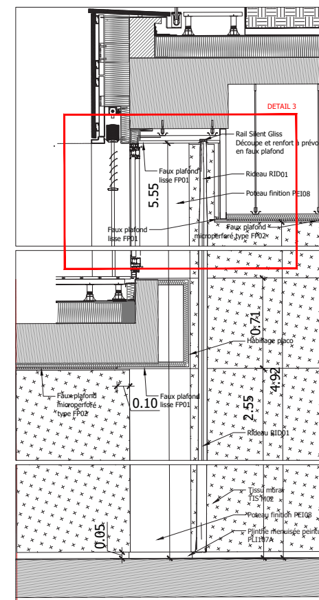
COUPE DD - 1/50 ème DETAIL 1007-1 GORGE LUMINEUSE - RIDEAU
