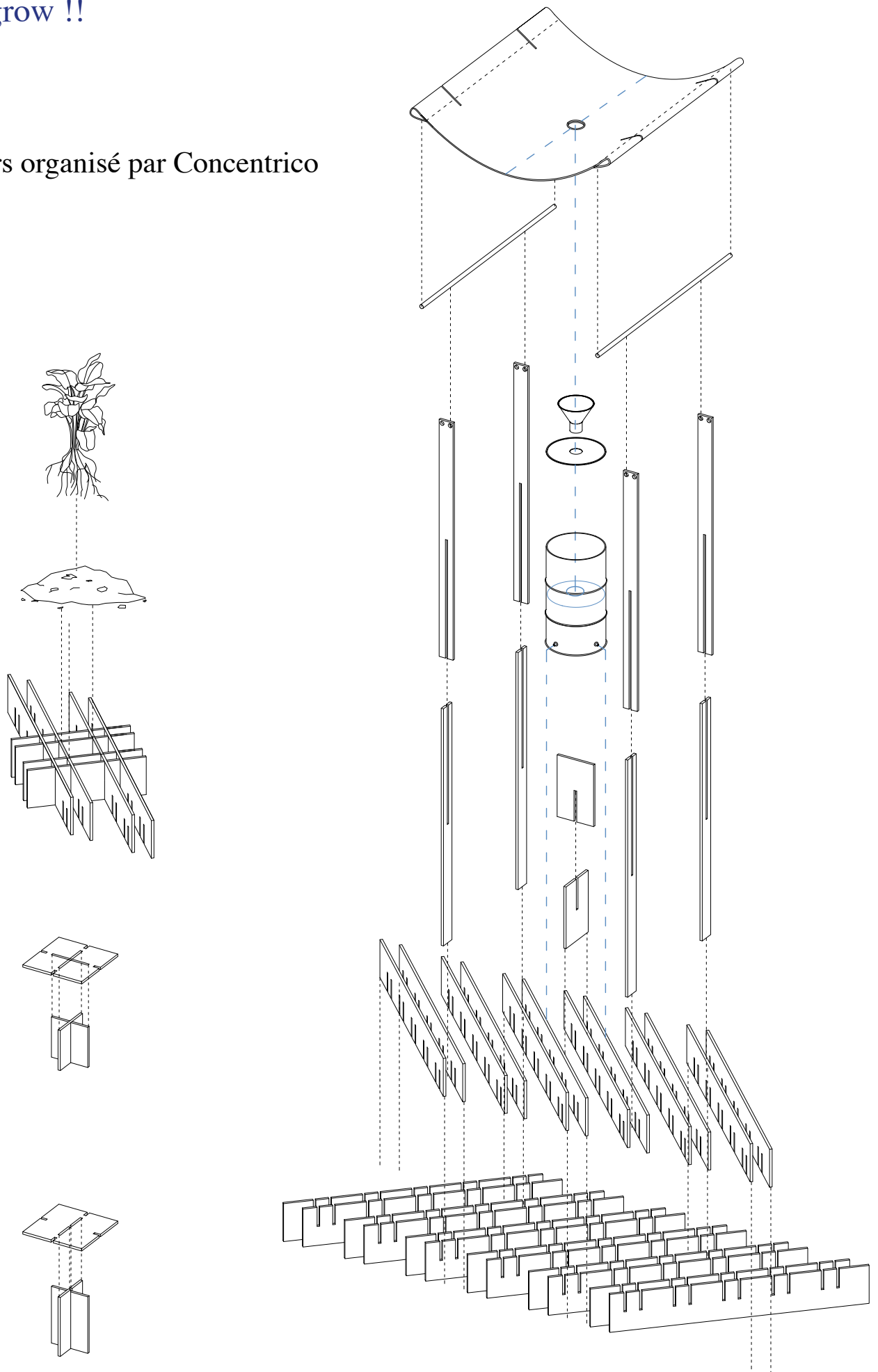
Axonométrie éclatée du système constructif de l'installation
