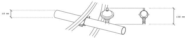
Détail anti-bélier inox à membrane 1/5
