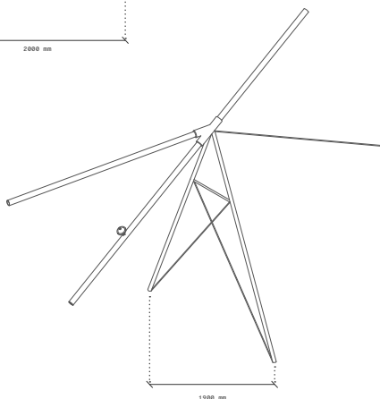
Axonométrie 1/20
