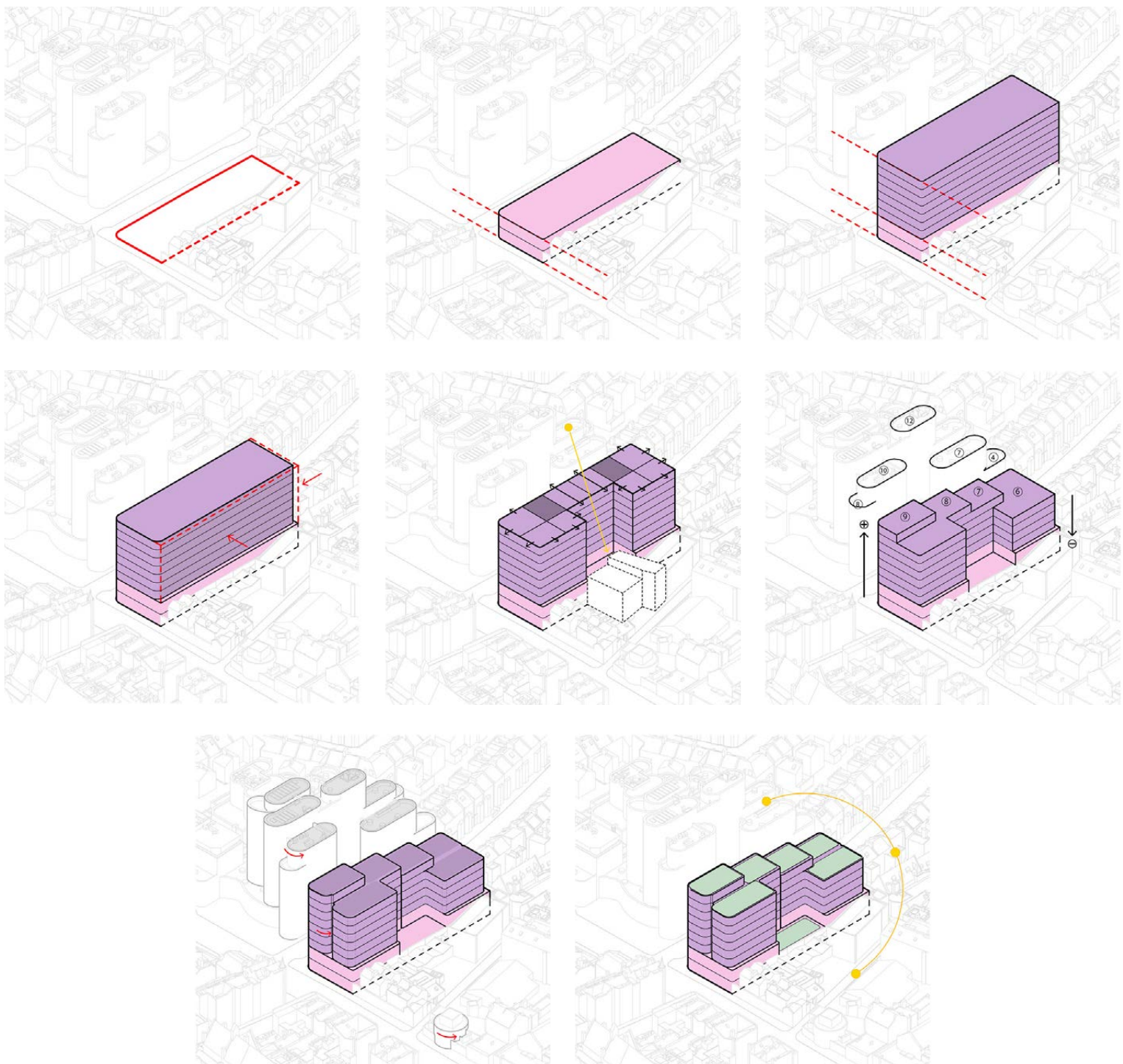
Schéma de définition du bâti
