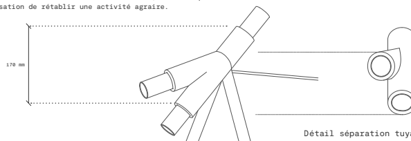
Détail séparation tuyau 1/5
