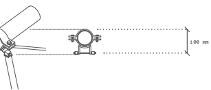
Détail fixation orientable 1/5
