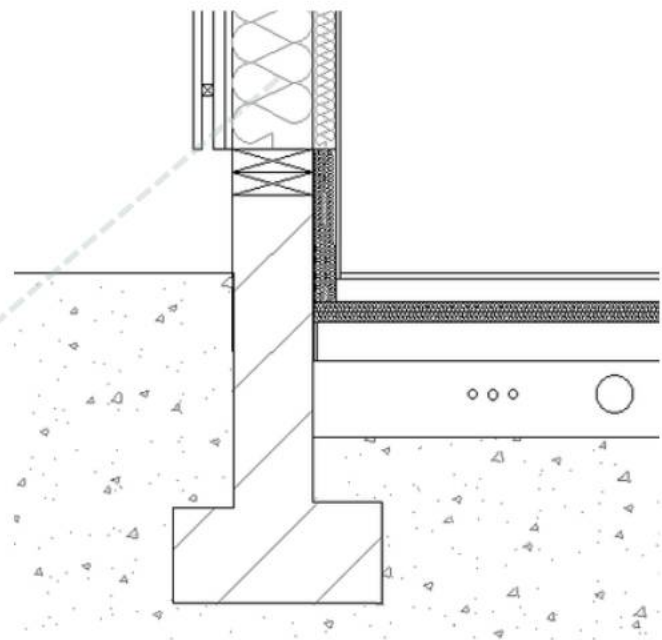
coupe technique - le moulin projet
