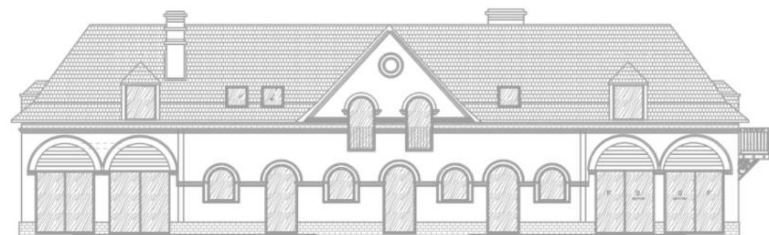
élévation nord - existant
