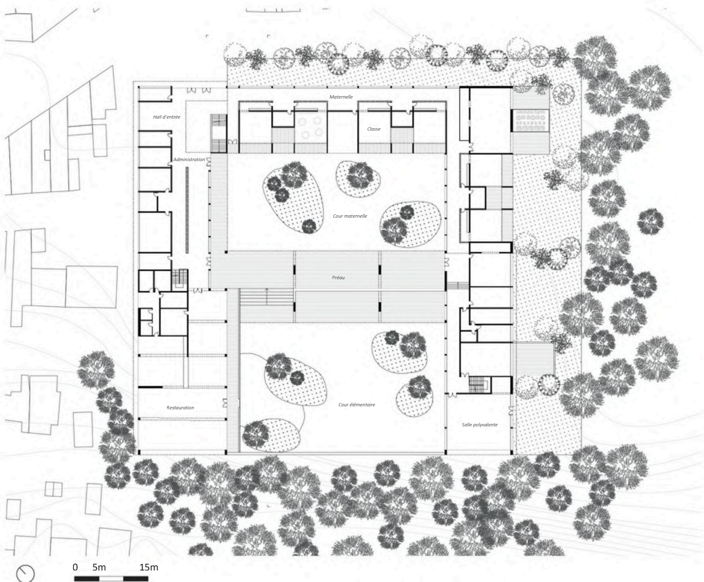
Plan du rez-de-chaussée
