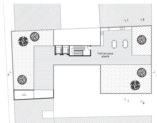
R+5 - Toiture-terrasse
