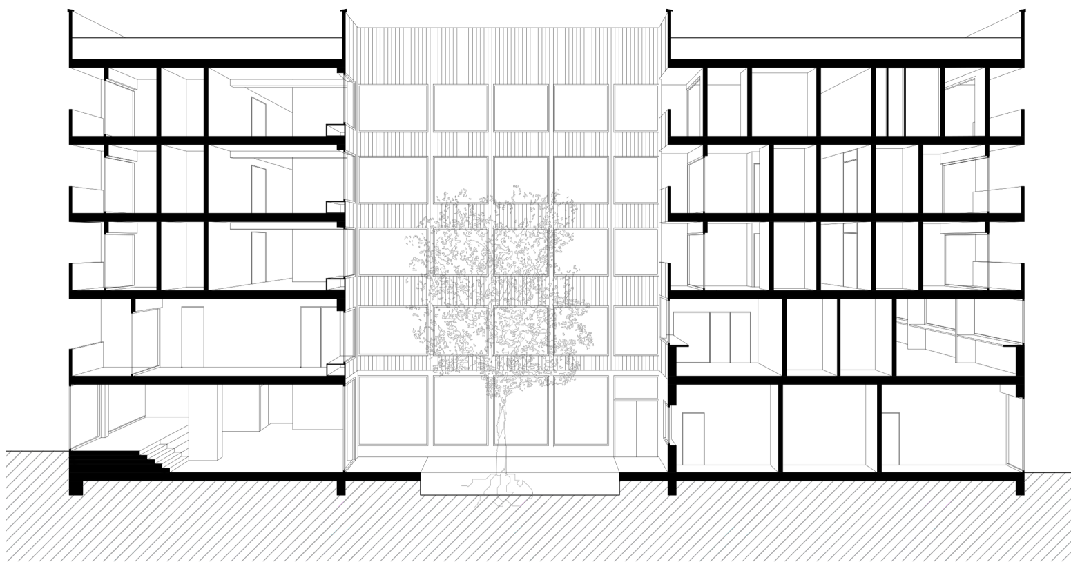
Coupe longitudinale sur le bâtiment
