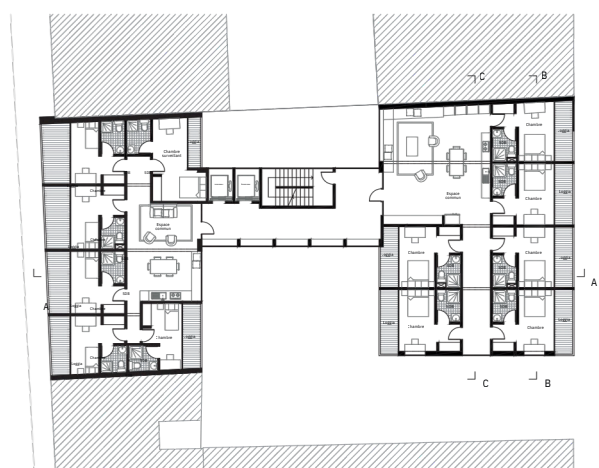
R+2
