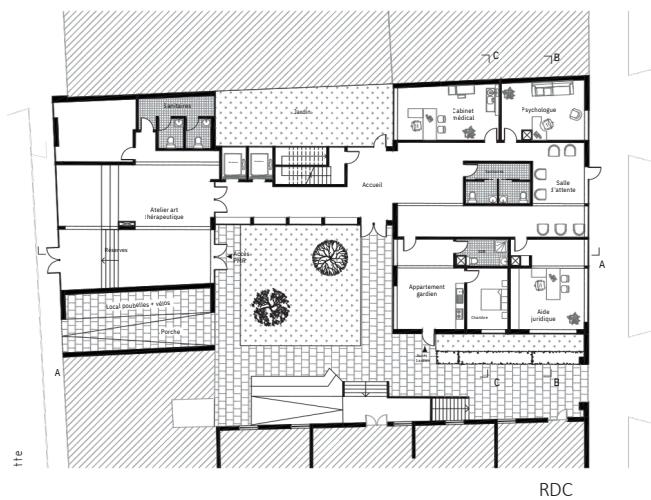
RDC
