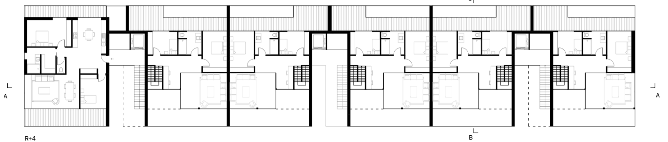
R+4
