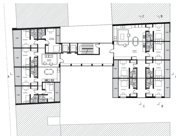
R+3
