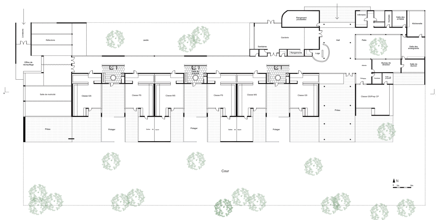
Plan de l'école
