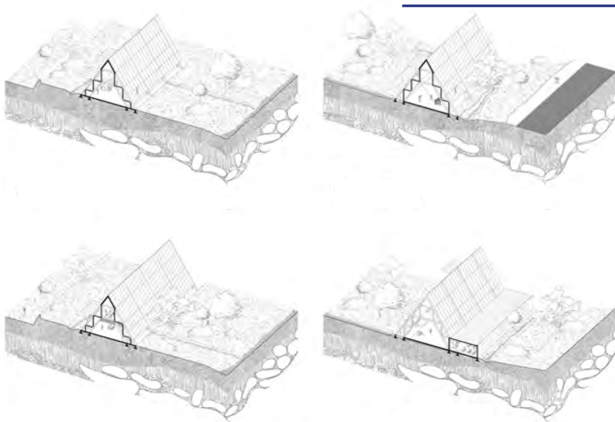
AXO | Coupe de différentes situation du système 1:200 Section of the different situations of the system 1:200
