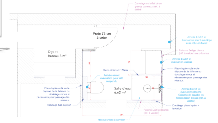
PLAN TECHNIQUE DU PROJET
