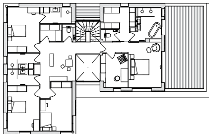
Premier étage
