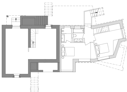
Sous-sol demi-enterré
