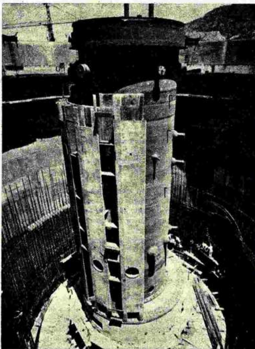
Reactor nuclear en fase de construcción. A pesar de su apariencia de solidez y seguridad, ha habido accidentes
