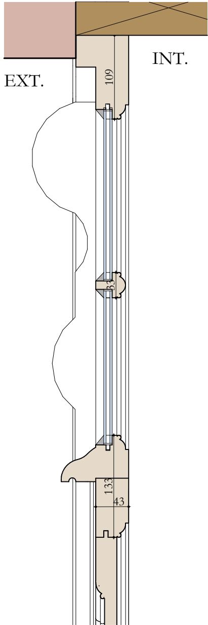
Section verticale DD
