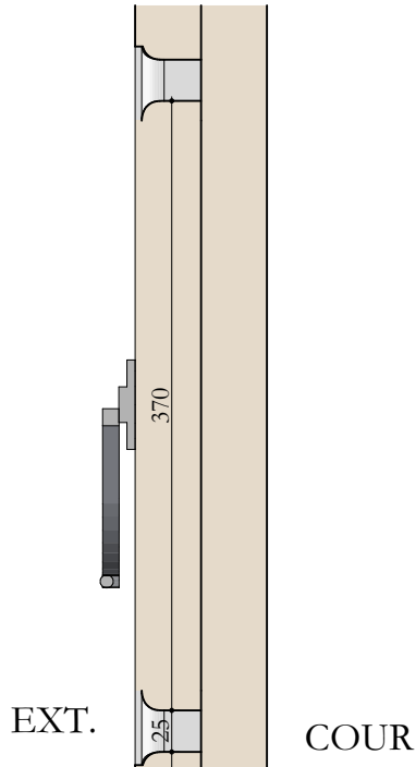
Section verticale DD
