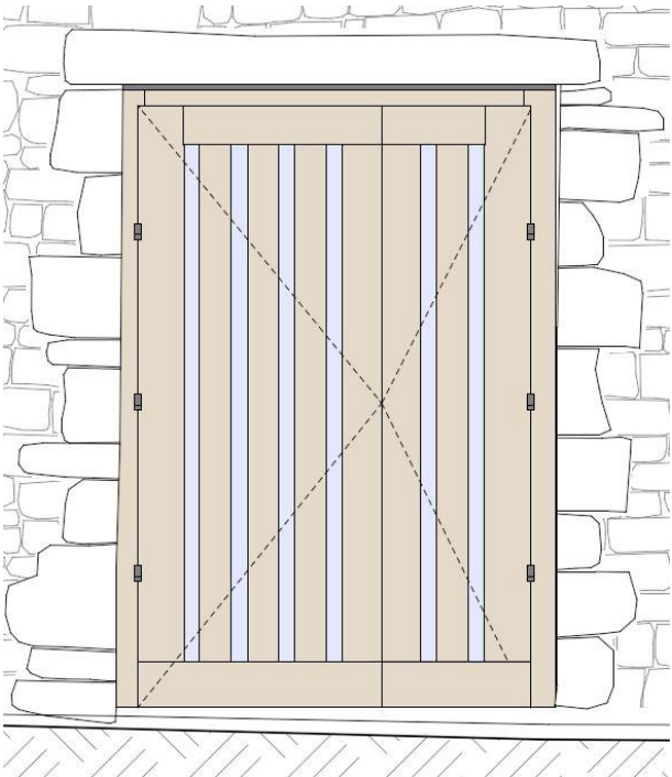
Dessin de la porte PO01 reconstituée – PROJET.
