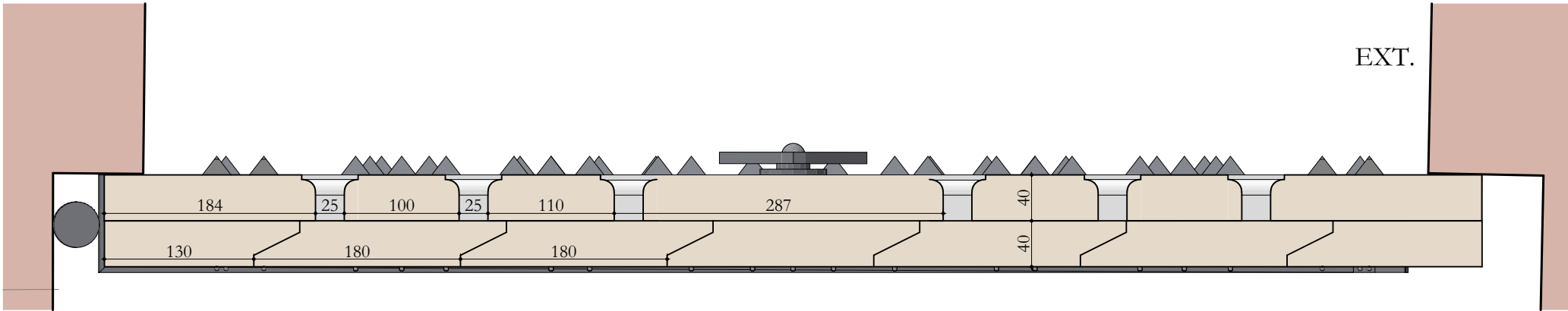
Section horizontale AA - Porte piétonne
