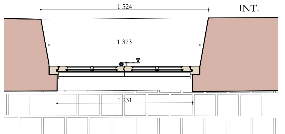
EXT. INT. Vue en plan
