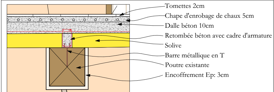
Détail 2 : projet plancher chauffant collaborant R+1 - 1/20°.
