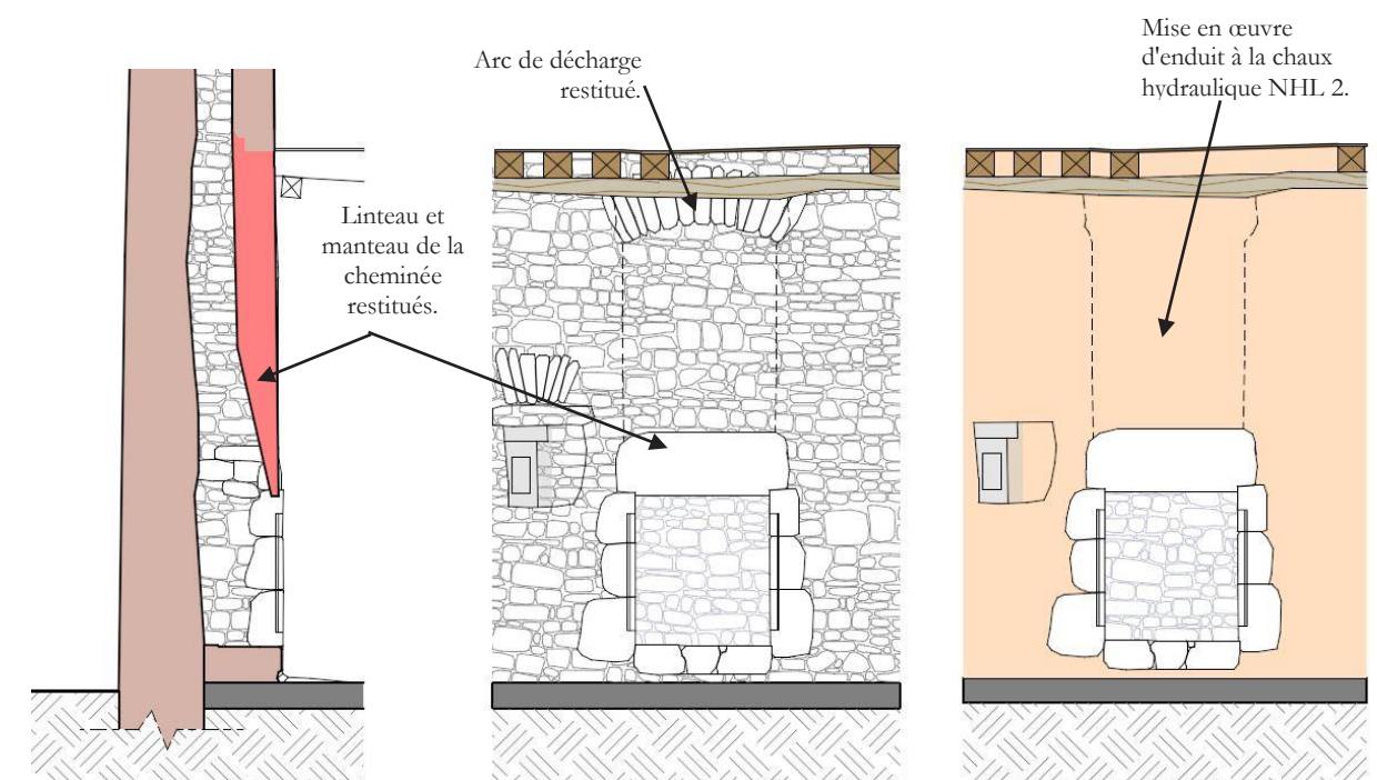
Schéma du projet de restauration de la cheminée de la tour sud-ouest.
