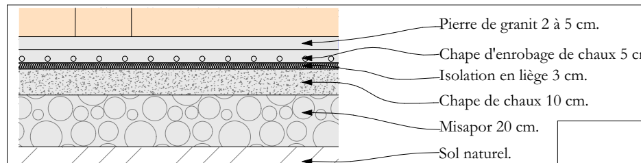
Détail 1 : projet de sol chauffant RDC - 1/20°.
