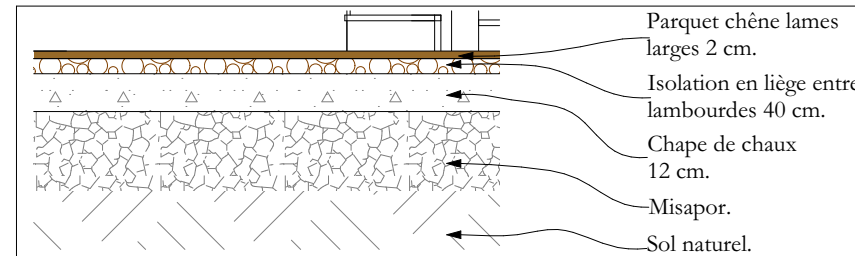
Détail 1 : projet de sol grand salon -1/20°.
