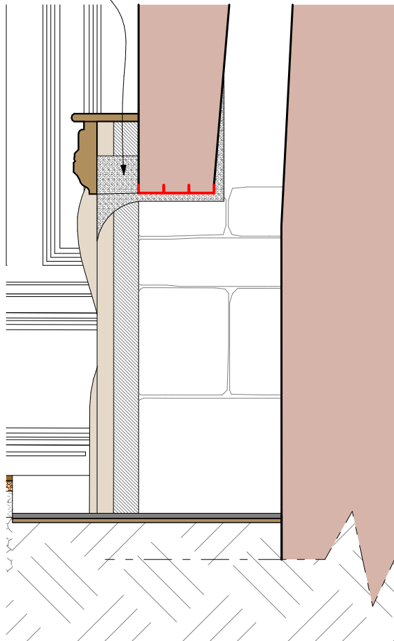
Détail sur le manteau de cheminée - Projet.
