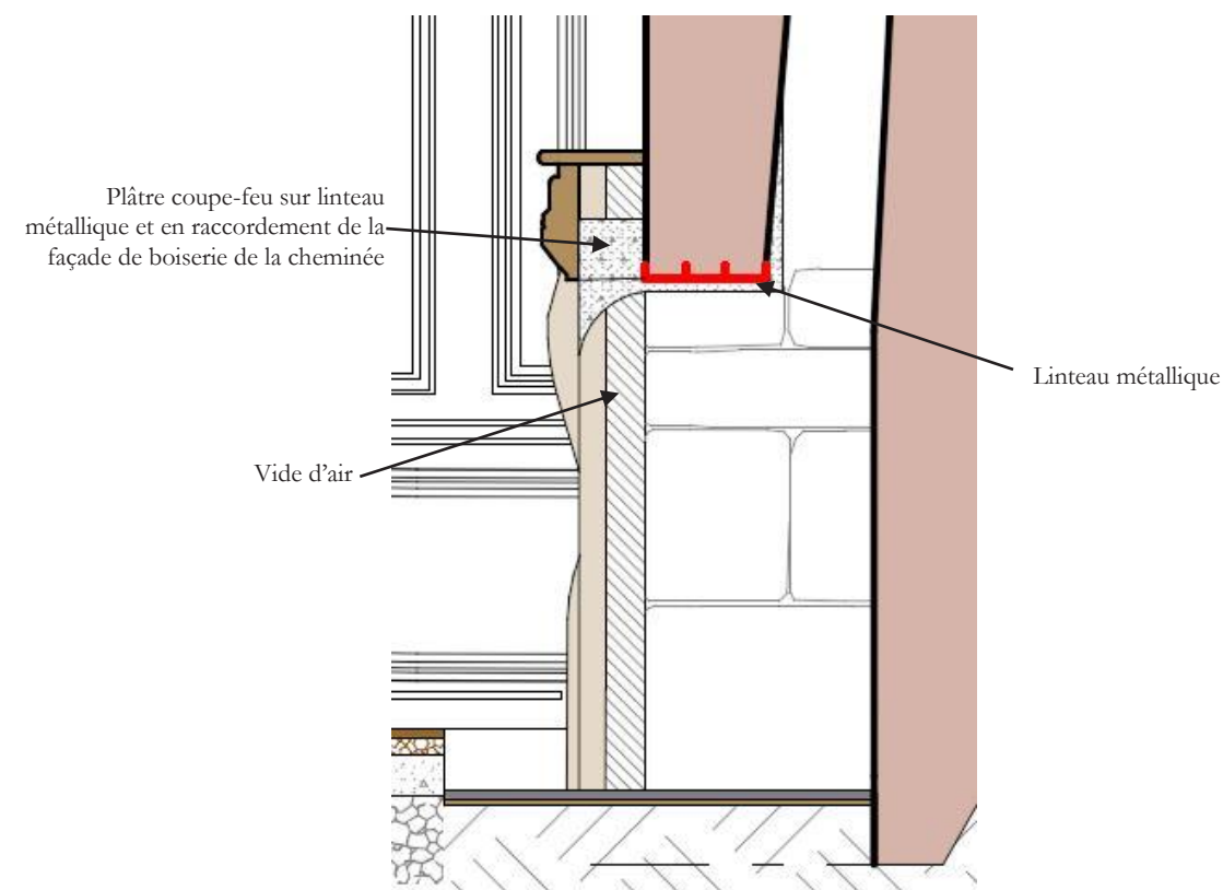
Détail du projet prévu sur la cheminée du grand salon.
