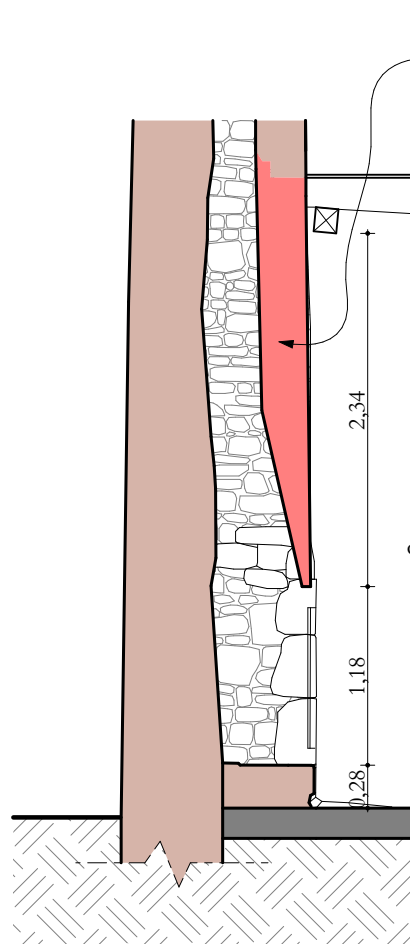
Cheminée de la tour sud-ouest future
