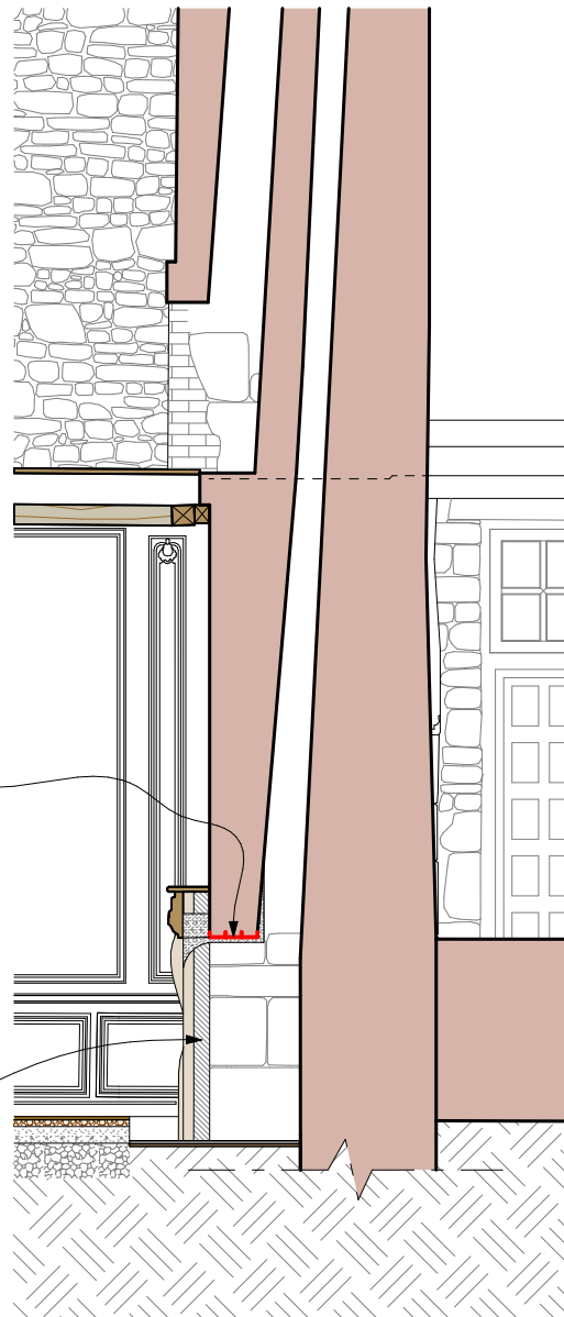
Coupe sur la cheminée du grand salon - Etat futur.
