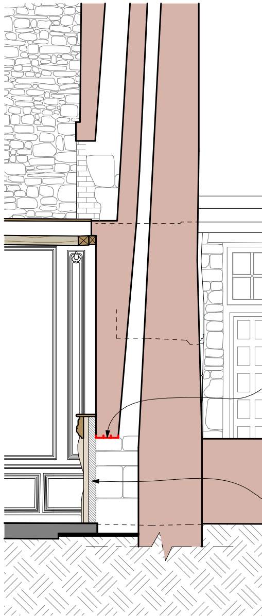
Coupe sur la cheminée du grand salon - Etat existant.
