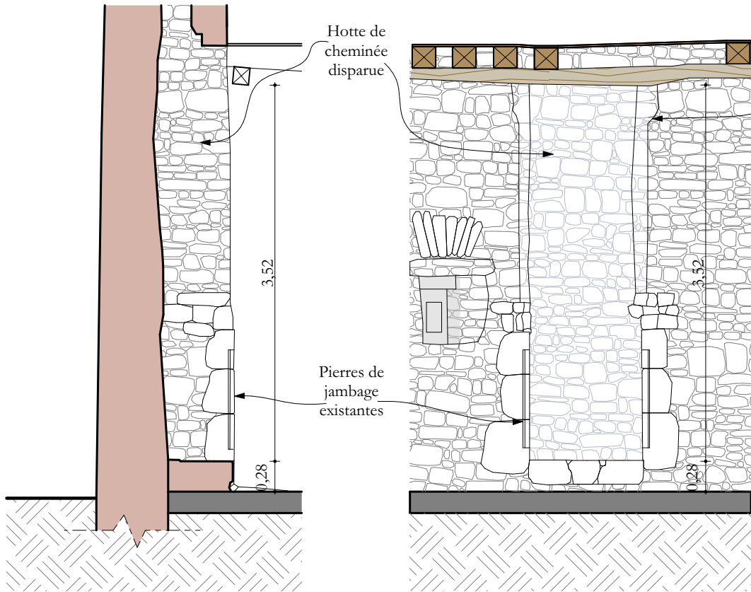
Cheminée de la tour sud-ouest existante
