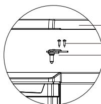
Tampa superior Parafuso de fixação Dobradiça superior
