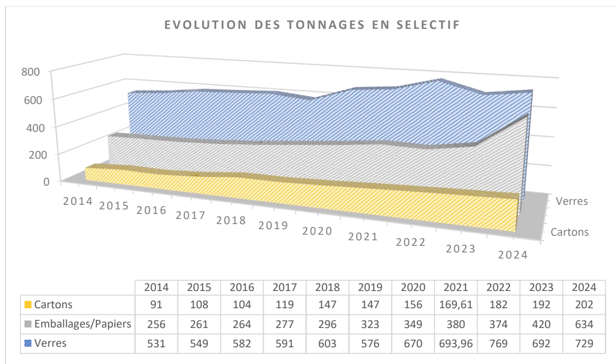
Figure 7 : évolution du tonnage des déchets recyclables
