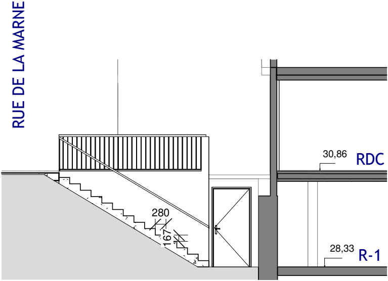
Coupe sortie B 1 : 100
