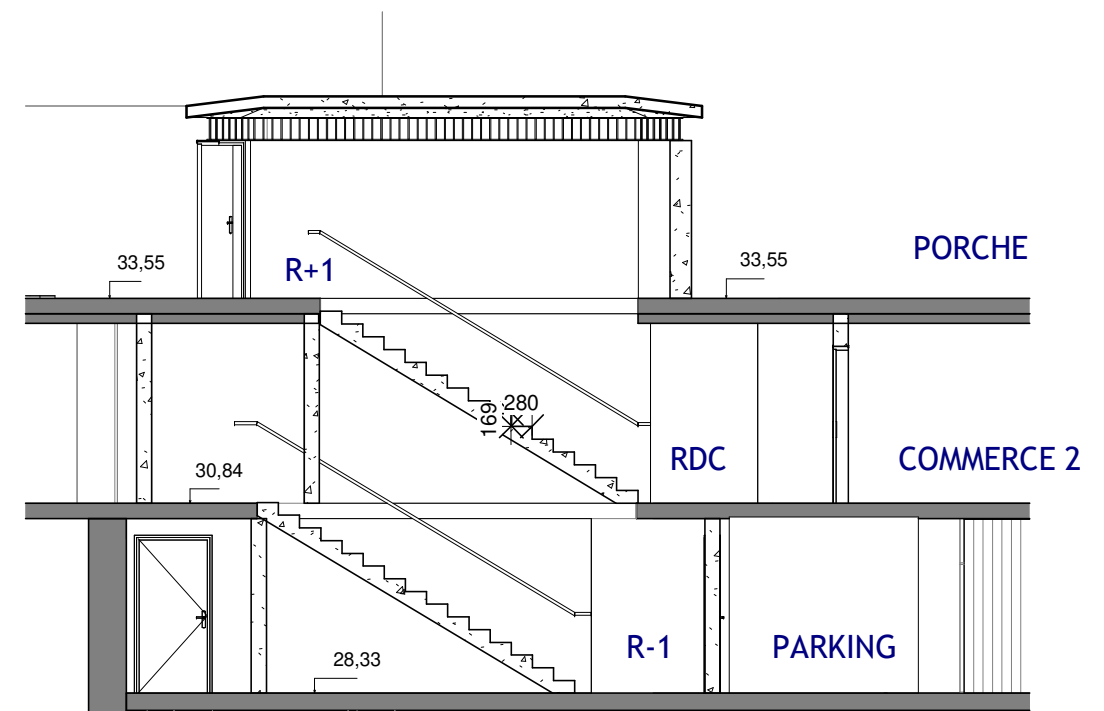
D2- Coupe Sortie D 1 : 100
