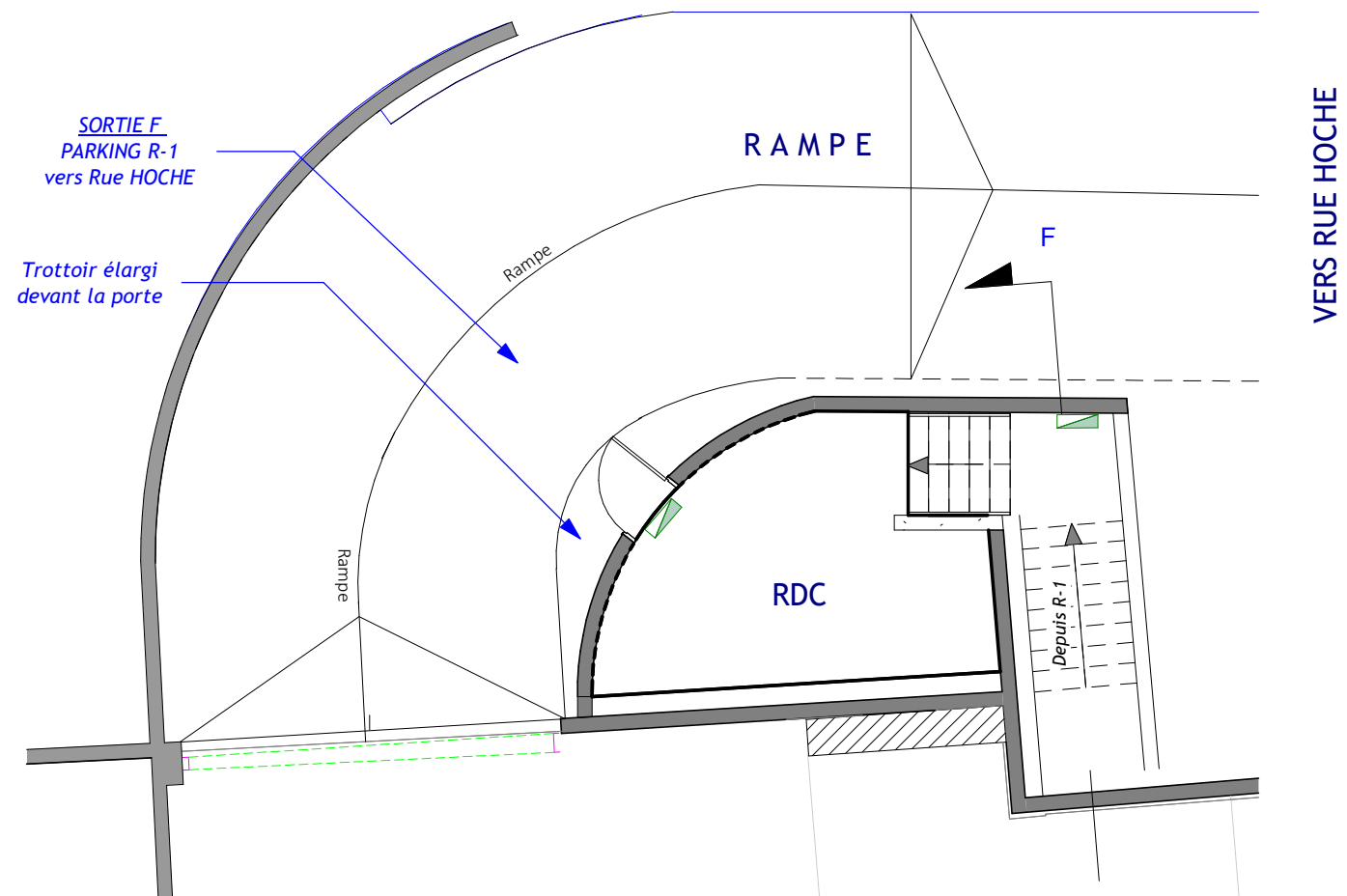
RDC Hoche PR - Sortie F 1 : 100
