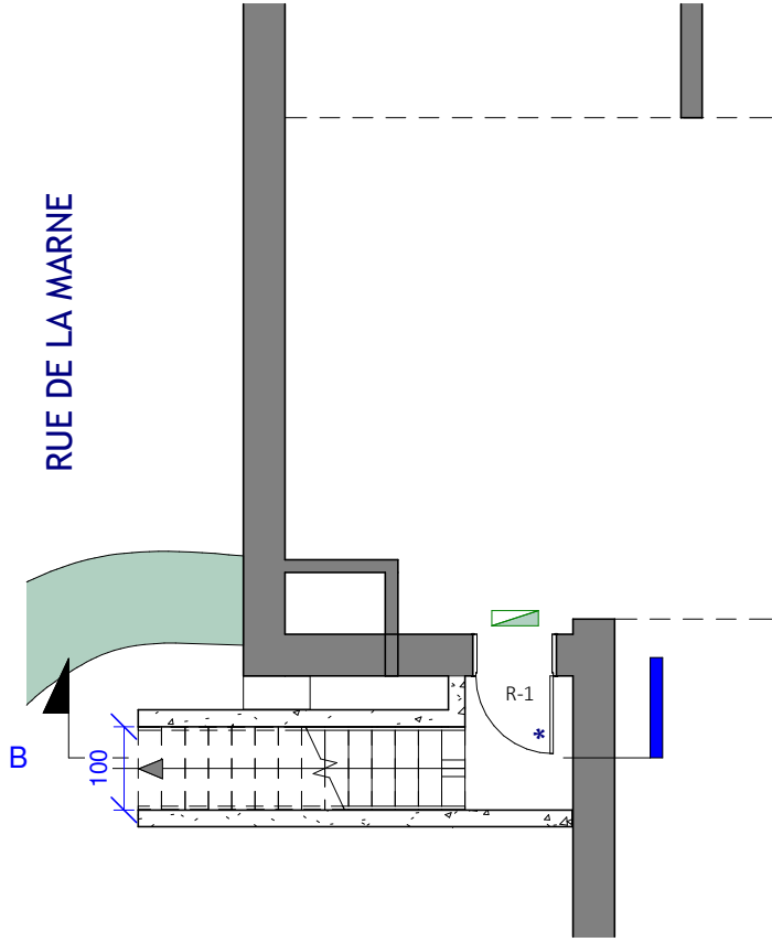
R-1 Marne PR - Sortie B 1 : 100
