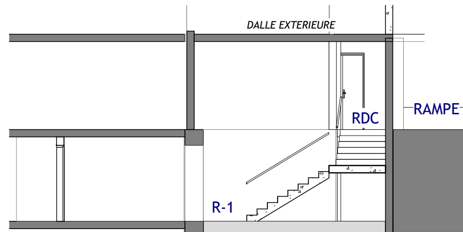
Coupe Sortie F 1 : 100
