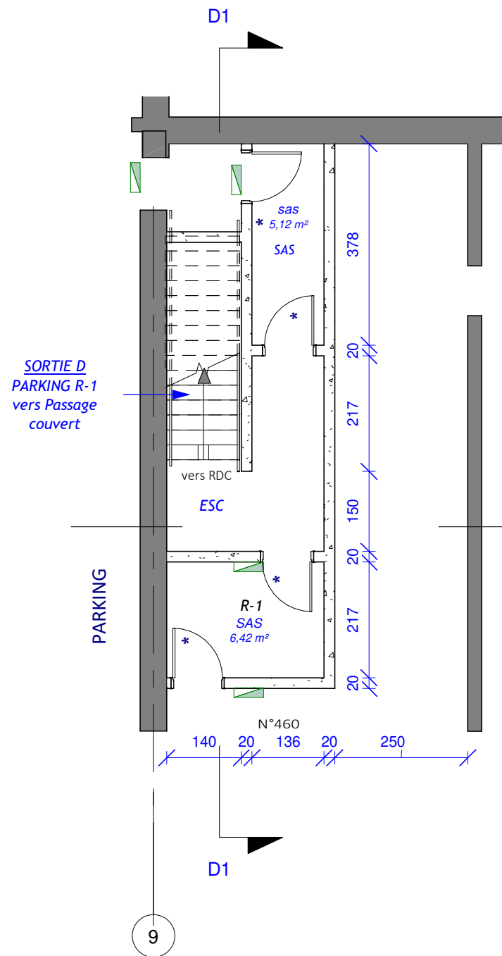
R-1 Marne PR - Sortie D 1 : 100
