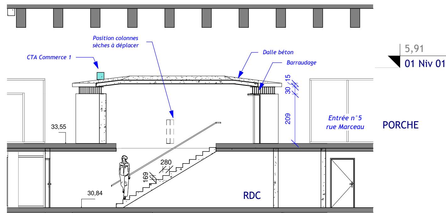
C1-Coupe Porche Sortie C 1 : 100
