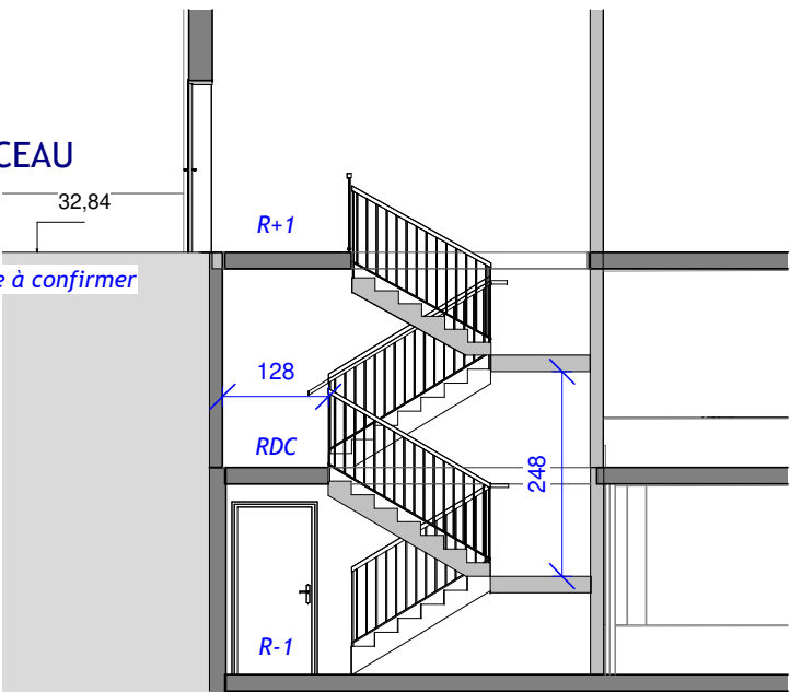
Coupe sortie E
