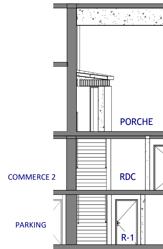
D2- Coupe Sortie D 1 : 100
